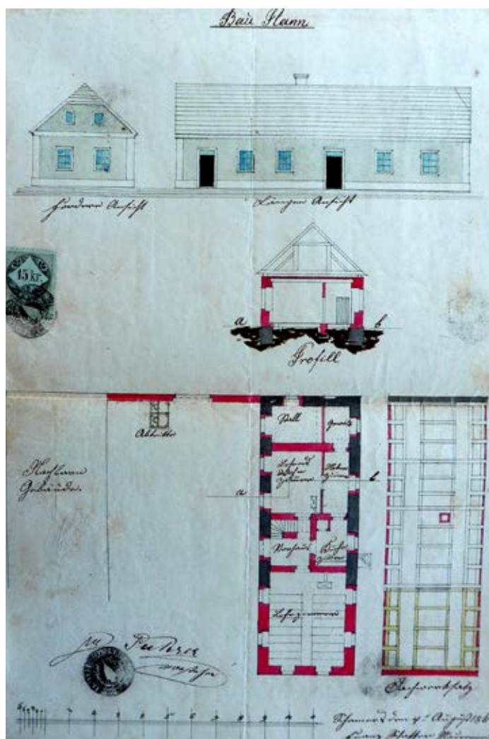
Obr. 10: Plán na rozšíření první školy v Nové Vsi z r. 1865 od J. Kocába
