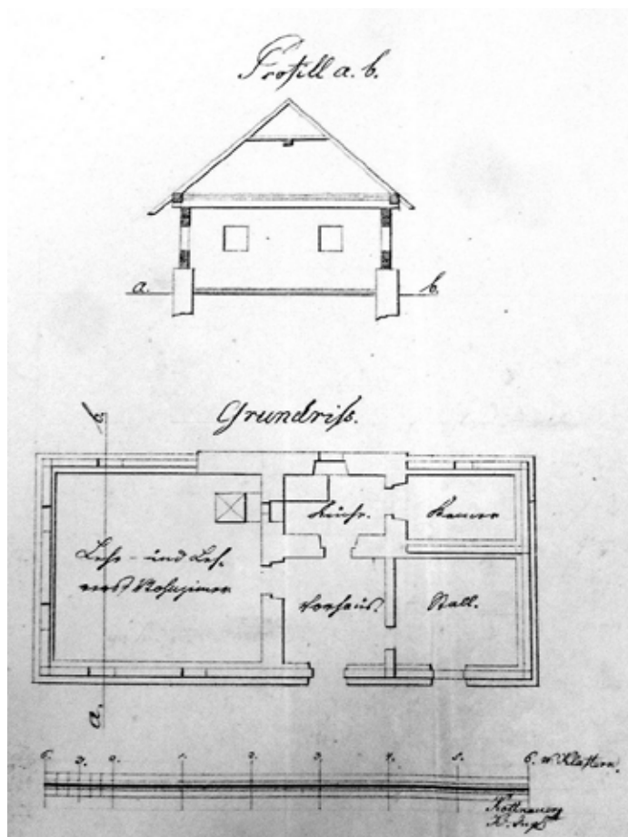
Obr. 6: Nejstarší srubová škola v Potočné na plánu z r. 1825
