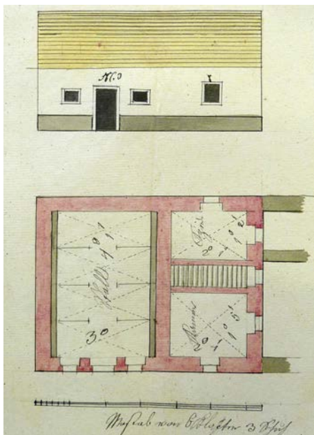
Obr. 5 Plán dostavby komory a chléva z r. 1836
